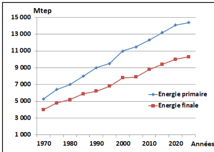
Figure 3 : Evolution de la consommation d'énergie primaire et finale dans le monde
