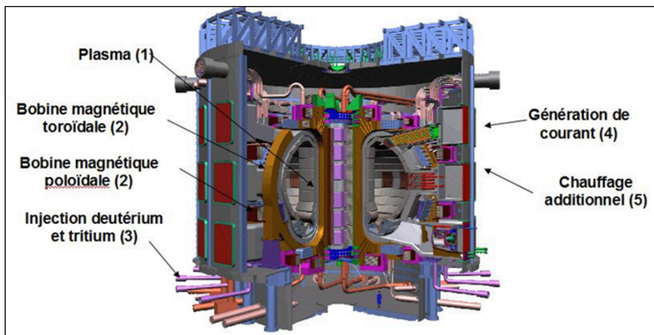
Figure 1 : Eclaté d'ITER
