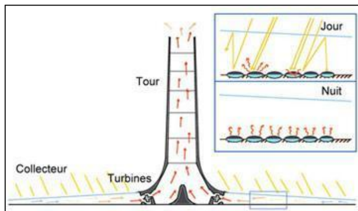
Figure 10 : Principe d'une centrale à effet de cheminée
