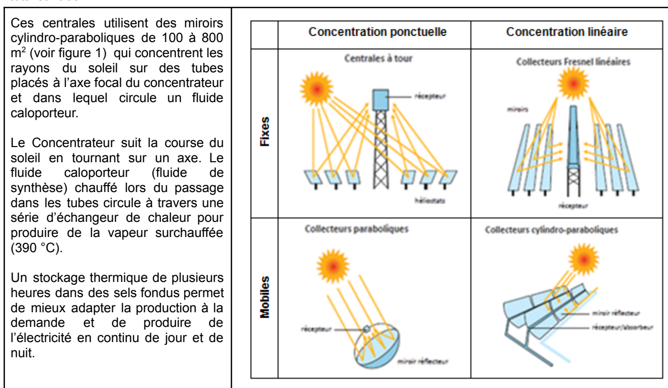
Figure 3 : Centrales à capteurs cylindro-paraboliques
