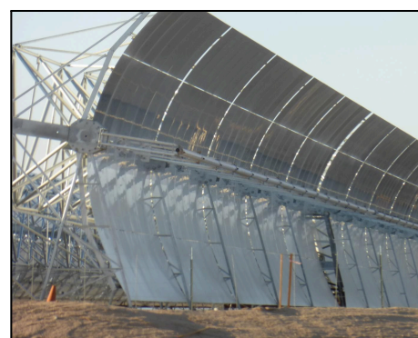
Figure 5 : Centrale de MOJAVE
