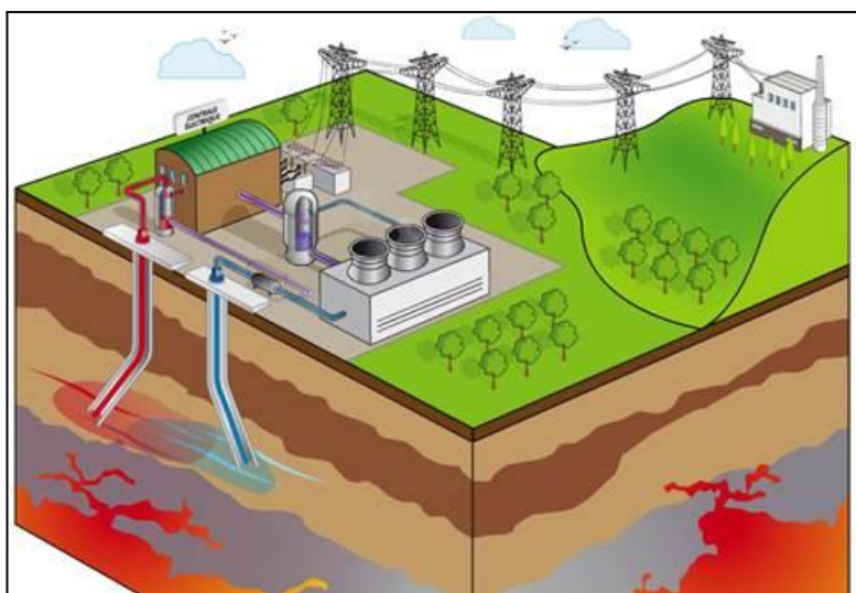
Centrale géothermique de Bouillante en Guadeloupe
