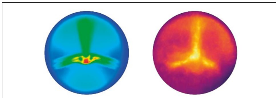
Imagerie X simulée (gauche) et expérimentale (droite) au démarrage des réactions de fusion
