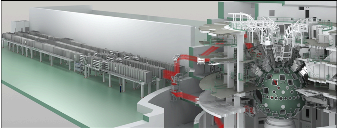
Chaînes laser et chambre d'expérience du LMJ
