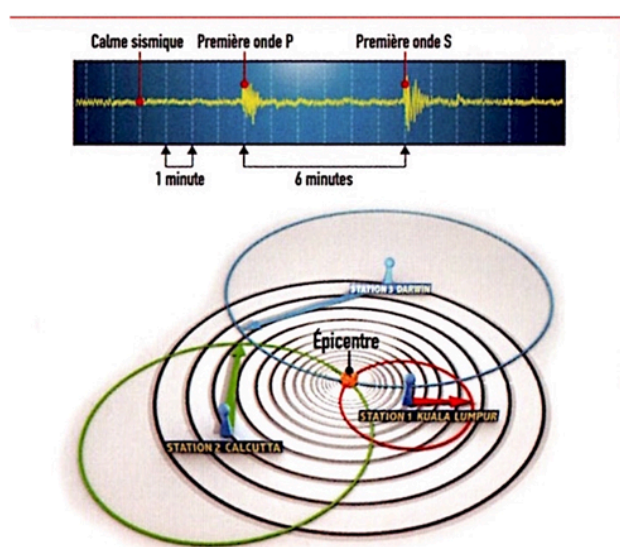
Figure 2 : Séisme de Sumatra enregistré par les stations de Calcutta, Kuala Lumpur et Darwin
