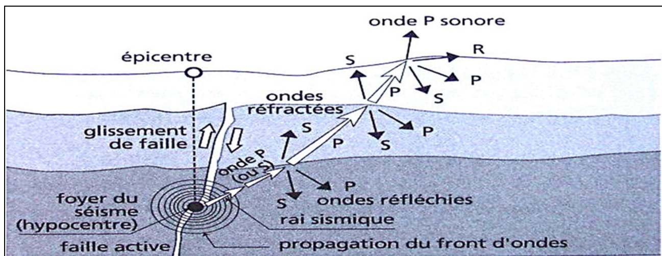
Figure 1 : Propagation des ondes sismiques
