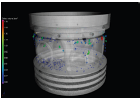
Caractérisation de porosité dans une pièce de fonderie par tomographie à rayons X
