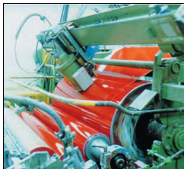
Mesure de grammage par rétrodiffusion © Source UARGA
