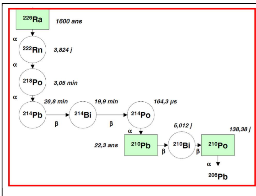
Figure 1 : Chaîne de désintégration du Ra 226 ►
