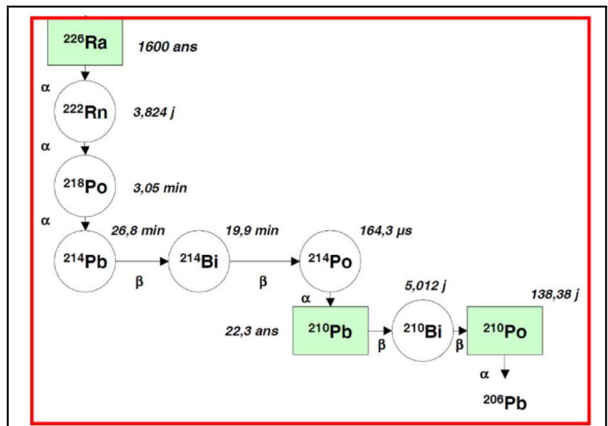
Figure 2 : Chaîne de désintégration du Radon 226 ►
